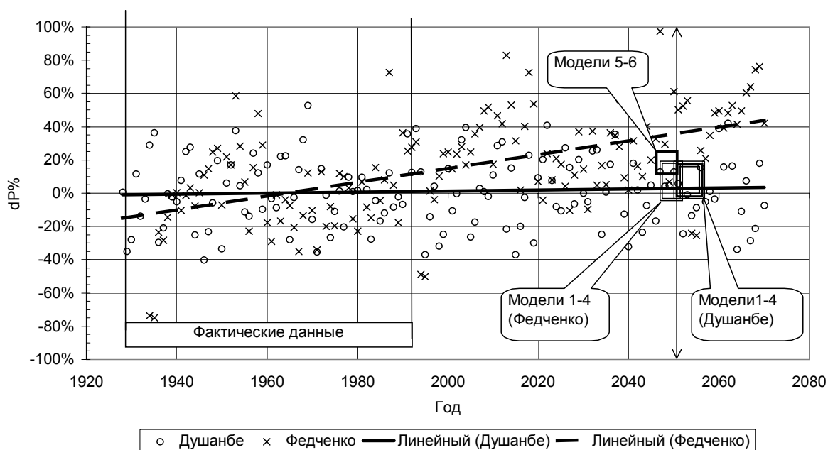
Рис. 3. Сравнение хронологического хода фактической суммы годовых осадков, прогностических данных по климатическим моделям пакета MAGICC (модели 1 – 4) и спектральному анализу для Душанбе и л. Федченко (модели 5 – 6). Показан линейный тренд спектральной прогностической оценки.
