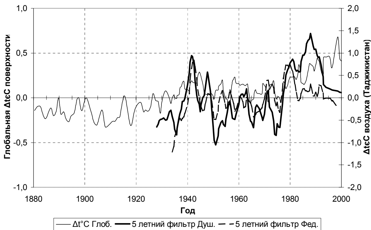
Рис. 1. Отклонение от нормы средней температуры поверхности Земного шара и температуры воздуха по данным двух станций Таджикистана.
