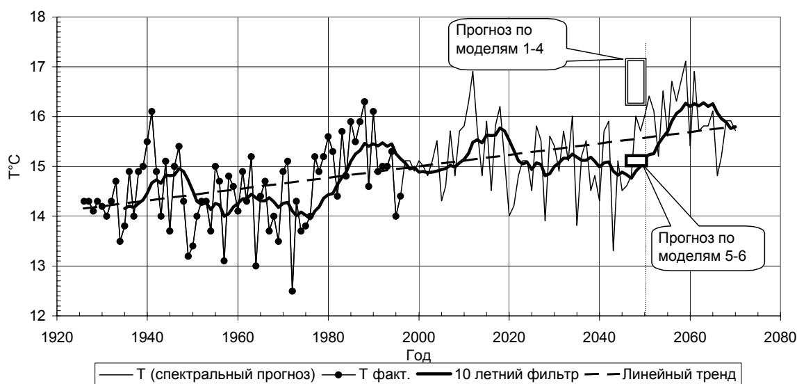
Рис. 2. Сравнение хронологического хода фактической среднегодовой температуры воздуха, прогностических данных по климатическим моделям пакета MAGICC (модели 1 – 4) и спектральному анализу для Душанбе (модели 5 – 6). Показан линейный и 10-летний скользящий тренды спектральной прогностической оценки.
